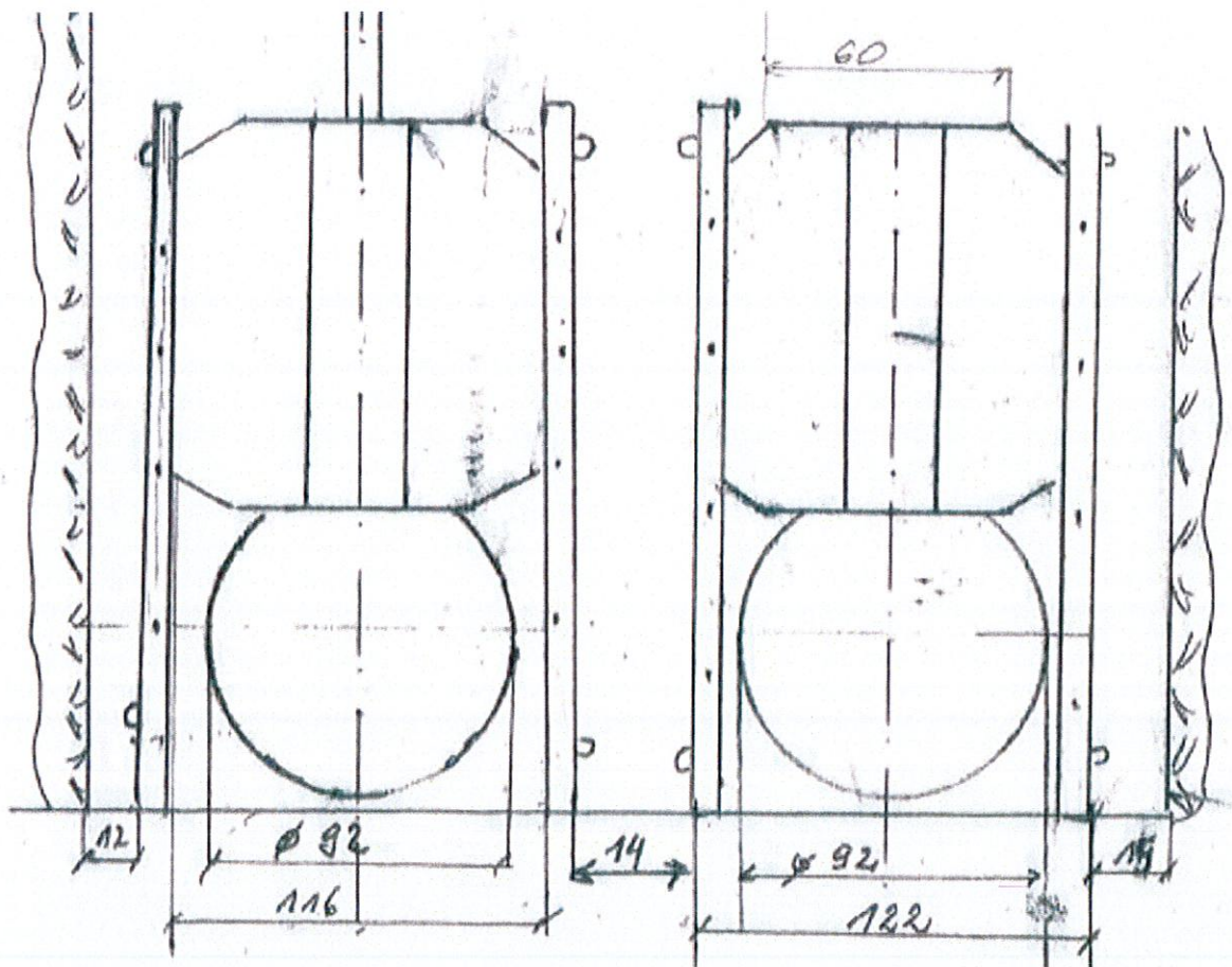
Rys. 1. Szkic zasuw
