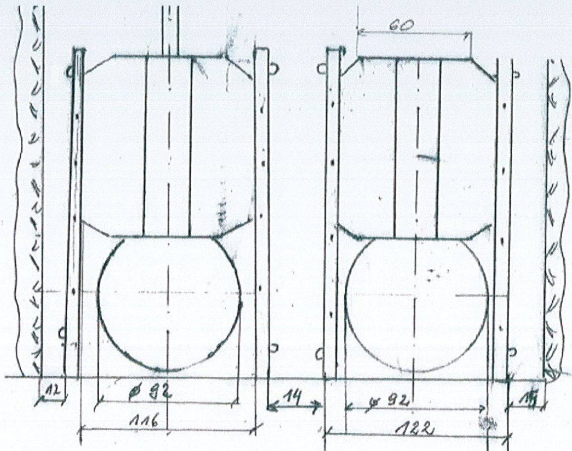
Rys. 1. Szkic zasuw
