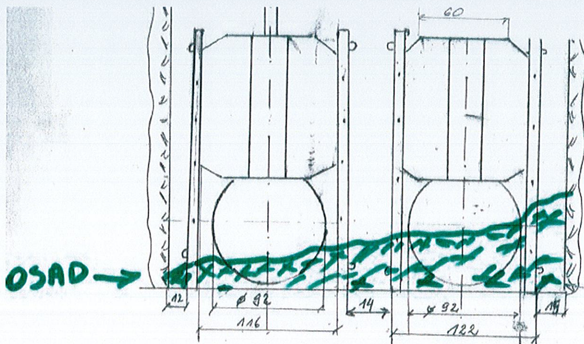
Rys. 4. Szkic zalegania osadu w komorze nr 2
