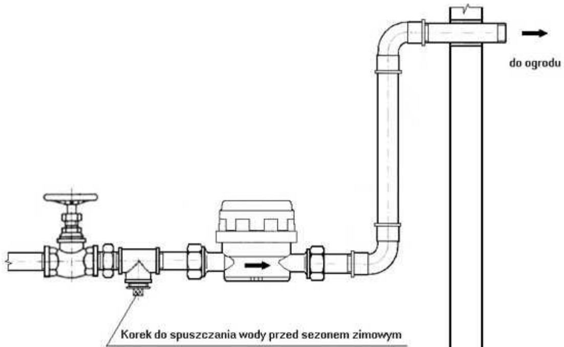
Przykładowa zabudowa podlicznika do podlewania ogrodu
