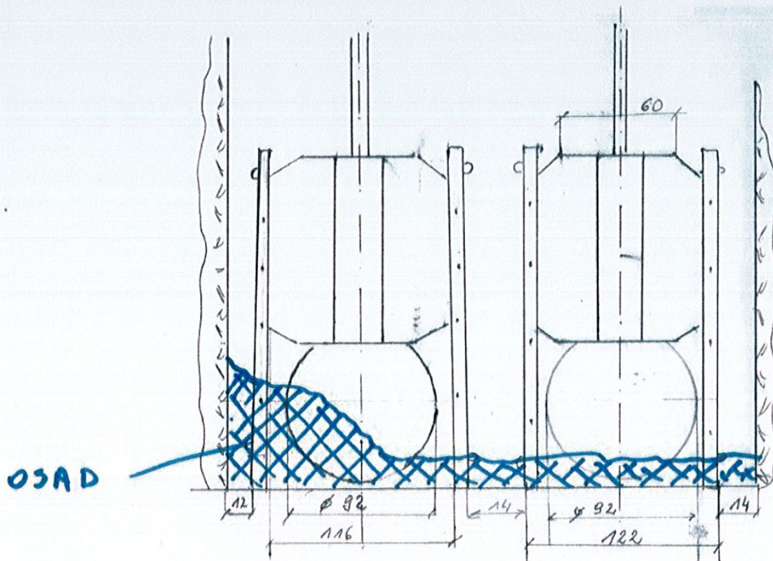
Rys. Szkic zalegania osadu w komorze nr 1
