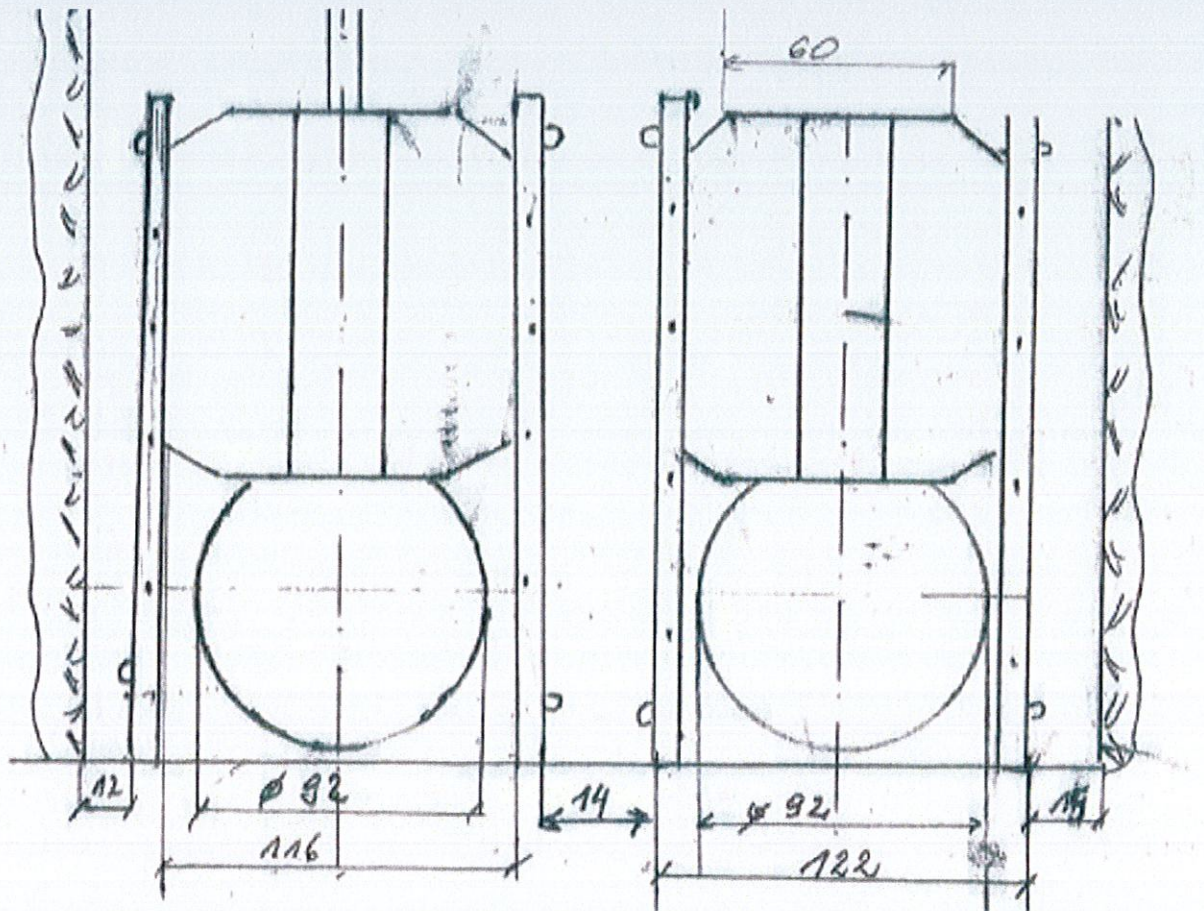
Rys. 1. Szkic zasuw
