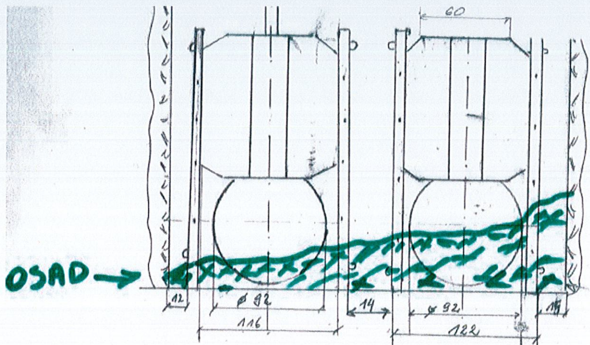
Rys. 4. Szkic zalegania osadu w komorze nr 2
