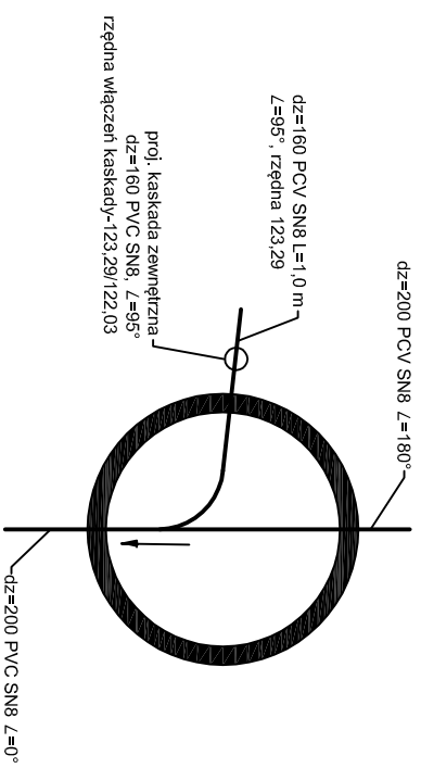
STUDNIA - S2 125,61/122,03 H=3,58 m
