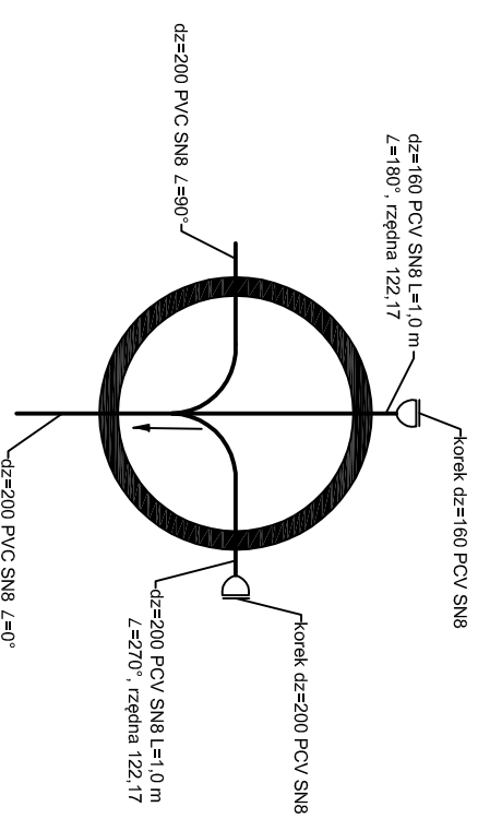
STUDNIA - S3 125,50/122,17 H=3,33 m
